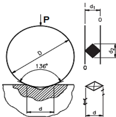
Figura 7: Desenho esquemático dos ensaios Brinell e Vickers.
